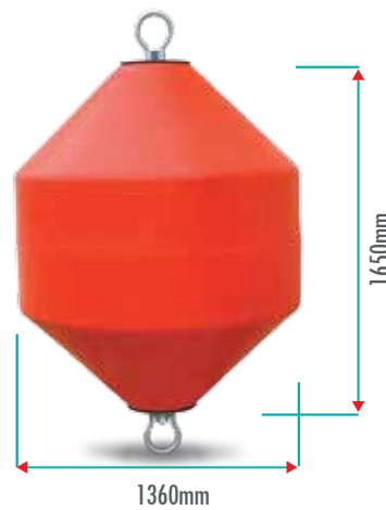
M03290 1600 LT ŞAMANDIRA / BUOY Yüzdürmesi / Buoyancy: 1500 kg Ürün Ağırlığı / Weight: 110 kg
